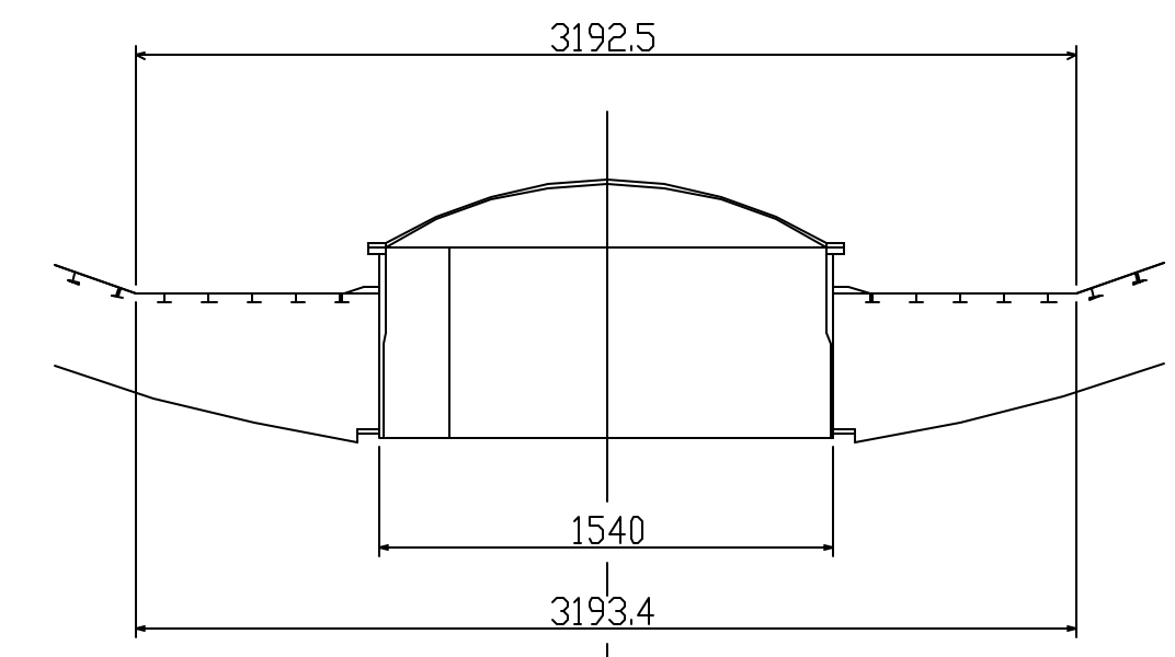
D-D
